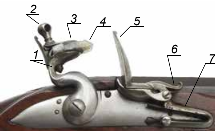
Кременевий замок: 1 – курок; 2 – курковий гвинт; 3 – верхня губа курка; 4 – кремій; 5 – кришка (кресало); 6 – полиця; 7 – підкресальна пружина
