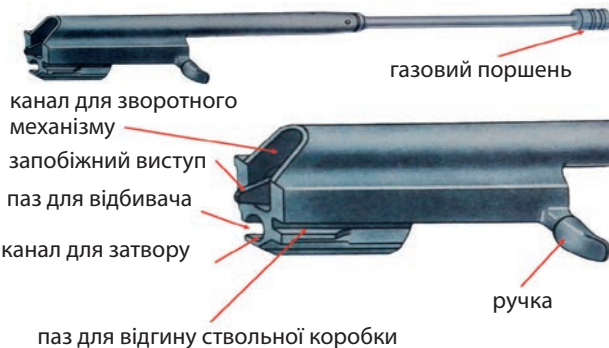
• Затворна рама з газовим поршнем
