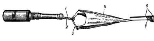
Іл. 3.7. Граната РКГ-3 під час польоту: 1 — пружина стабілізатора; 2 — рухома трубка; 3 — дротяні п'р'їни; 4 — матер'яний конус; 5 — відкидний ковпак з планкою; 6 — пружина ковпака
