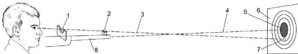
Іл. 2.8. Схема прицілювання в разі перевищення середньої точки прицілювання: 1 — середина прорізу прицілу; 2 — верхній край мушки; 3 — лінія прицілювання; 4 — середня траєкторія куль; 5 — середня точка влучення — центр мішені; 6 — мішень; 7 — точка прицілювання; 8 — ствол гвинтівки
