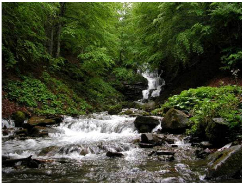
Рис. 49. Звір – вузька, глибоковрізана V-подібна долина з потоком
