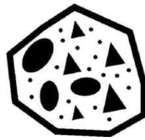
Моренні пасма
