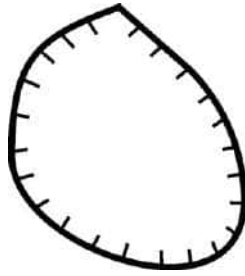
Водозбірні лійки
