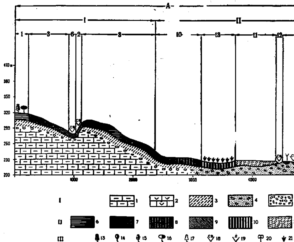
Рис. 1 . Ландшафтний профіль (за Г. П. Міллером, Г. Г. Моголо I — геологічна основа: 1 — мерелі; 2 — гіпсоангідрити; 3 — лесовидні суглинки; 4 — азювіальні сугл II — ґрунти: 6 — дерново-підзолисті; 7 — сірі опідзолені; 8 — чорноземи опідзолені; 9 — перехідно-ка III — рослинність: 13 — дуб; 14 — граб; 15 — ія; 16 — сіровільшники; 17 — ліщина; 18 — різнотрав'я; 19 — осока; 20 — різнотрав'я; 21 — осока; 22 — і
