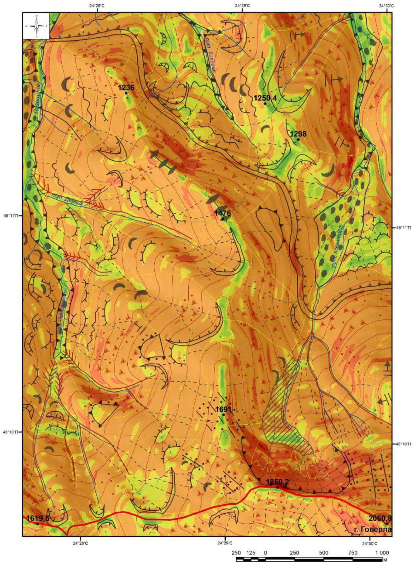
Рис. 42. Геоморфологічна карта басейну річки Лазещина
