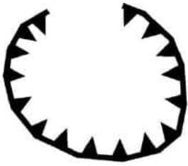
Давньольодовикові кари
