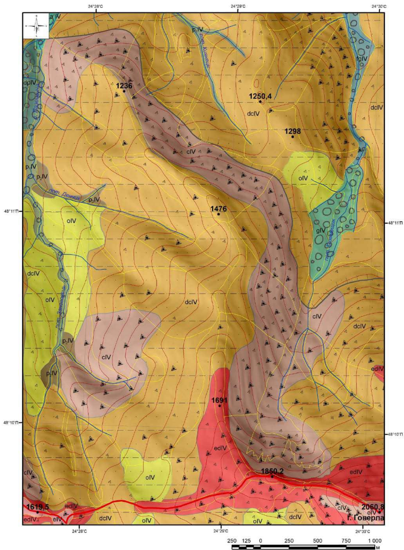
Рис. 40. Четвертинні відклади басейну річки Лазещина
