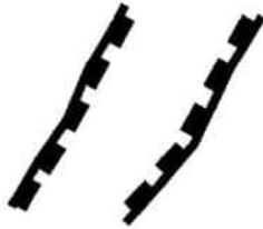
Трогові долини
