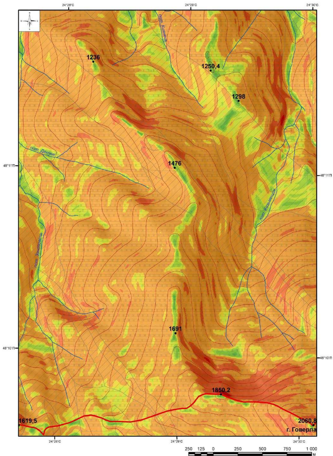
Рис. 41. Кругість схилів у басейні річки Лазещина
